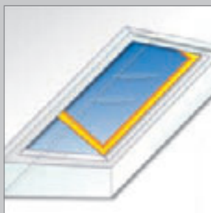
Wohndachausstieg WDA , Flügel wahlweise links oder rechts angeschlagen
