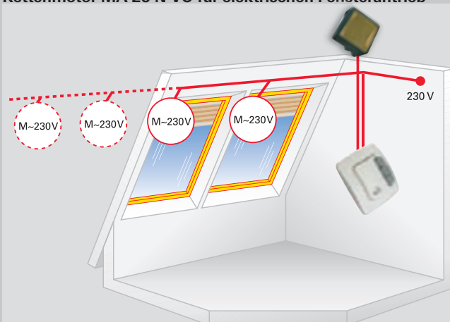
Kettenmotor MA 25 N VO für elektrischen Fensterantrieb
