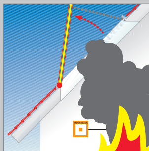
Rauch- und Wärmeabzugs-wohndachfenster WRA , optimaler Rauchabzug durch unten angeschlagenen Flügel
