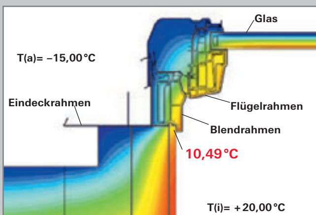
Isothermenverlauf ohne Wärmedämmung
