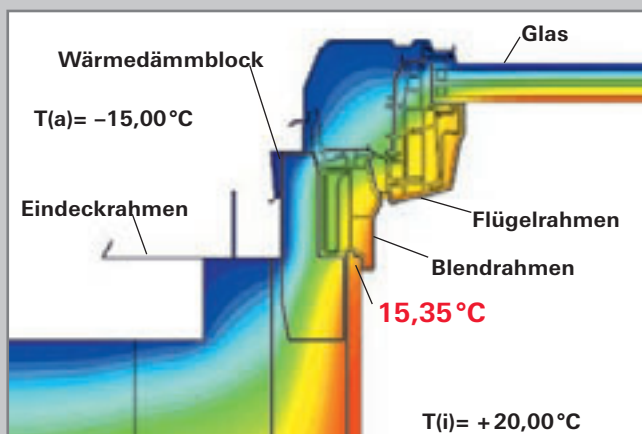
Isothermenverlauf eines Wohndachfensters 849 K mit Wärmedämmung
