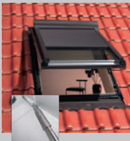
Außenrollladen Roto Therm: Beim Roto Therm manuell erfolgt die Bedienung über eine innen liegende, abnehmbare Handkurbel. (Außenoptik unterschiedlich zum Außenrollladen E.)
